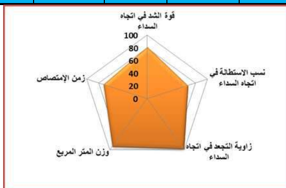
شكل (٧) معامل الجودة الكلية لأقل العينات المنتجة محل البحث
